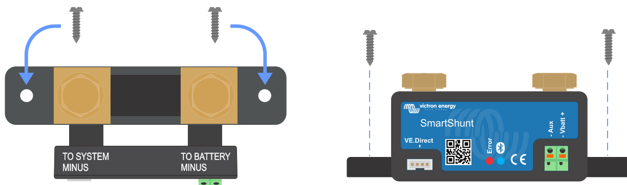
Bild ovanifrån på Smartshunt som visar monteringshålen och en sidobild av Smartshunt som visar monteringsmetod
