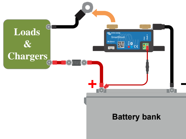
Utförande av en nollströmskalibrering
